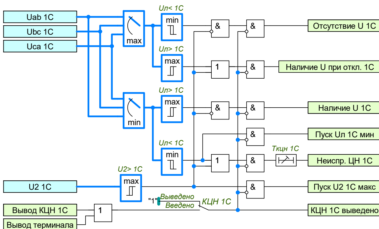
Рисунок 0.6 – Функциональный блок КЦН
