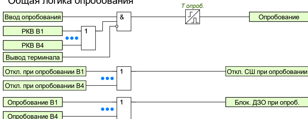
Рисунок 0.7 – Функциональный блок логики опробования
