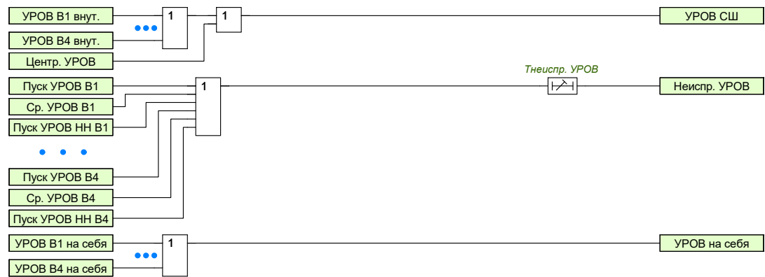
Рисунок 0.10 – Функциональный блок УРОВ СШ
