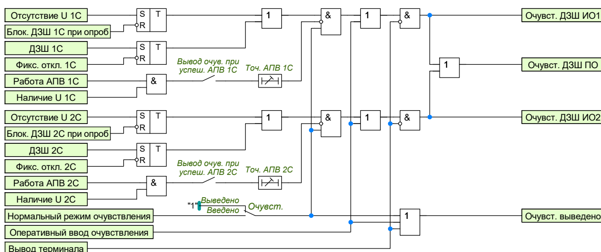
Рисунок 0.8 – Функциональный блок логики очувствления
