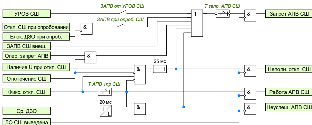
Рисунок 0.12 – Функциональный блок логики отключения СШ
